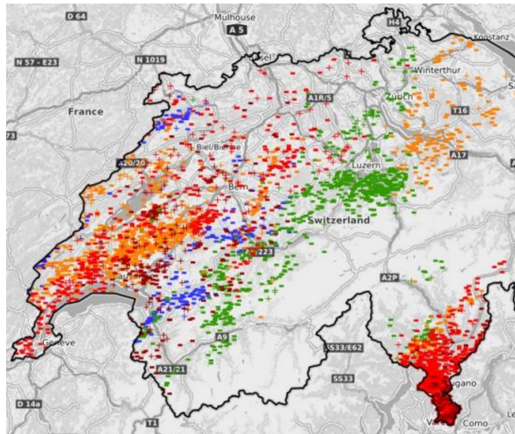
Attività dei fulmini (fulmini nuvola-terra CG) in Svizzera tra il 7 settembre alle ore 14:00 e l'8 settembre alle ore 02:00
